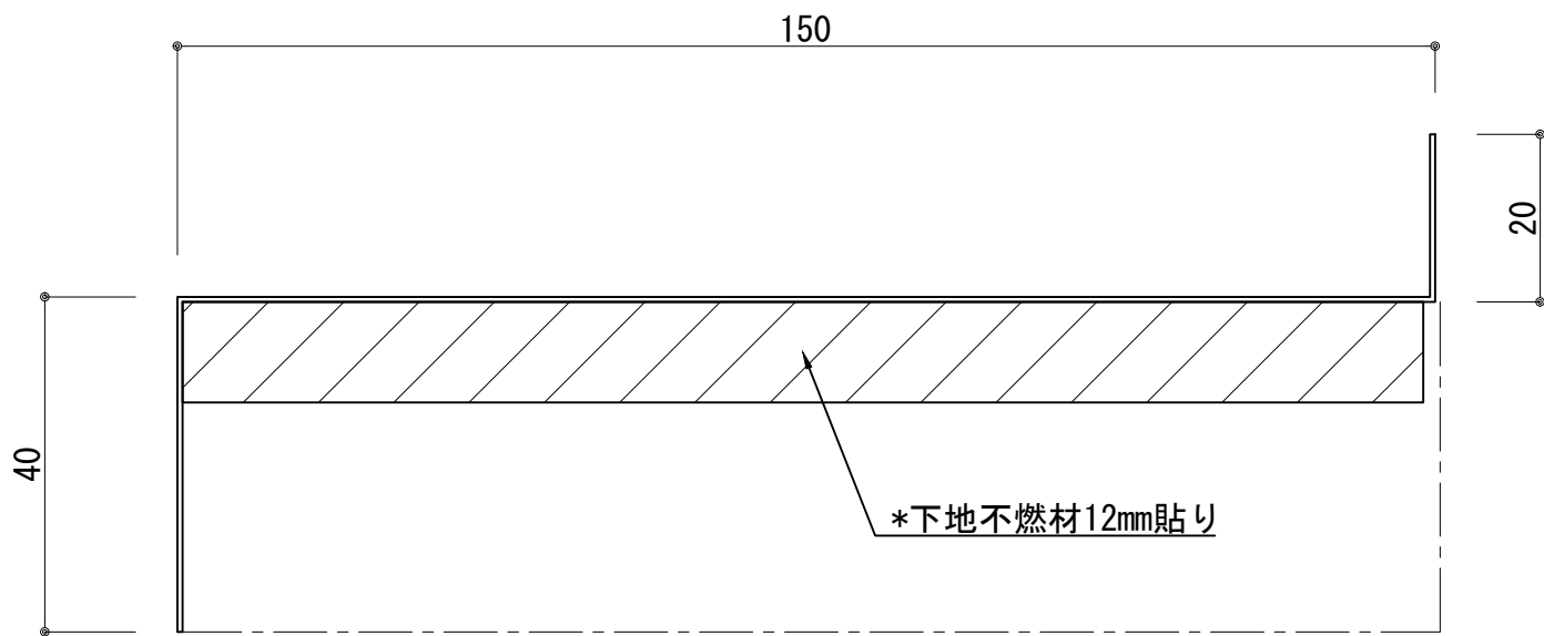
A-A'部断面図 1/1
