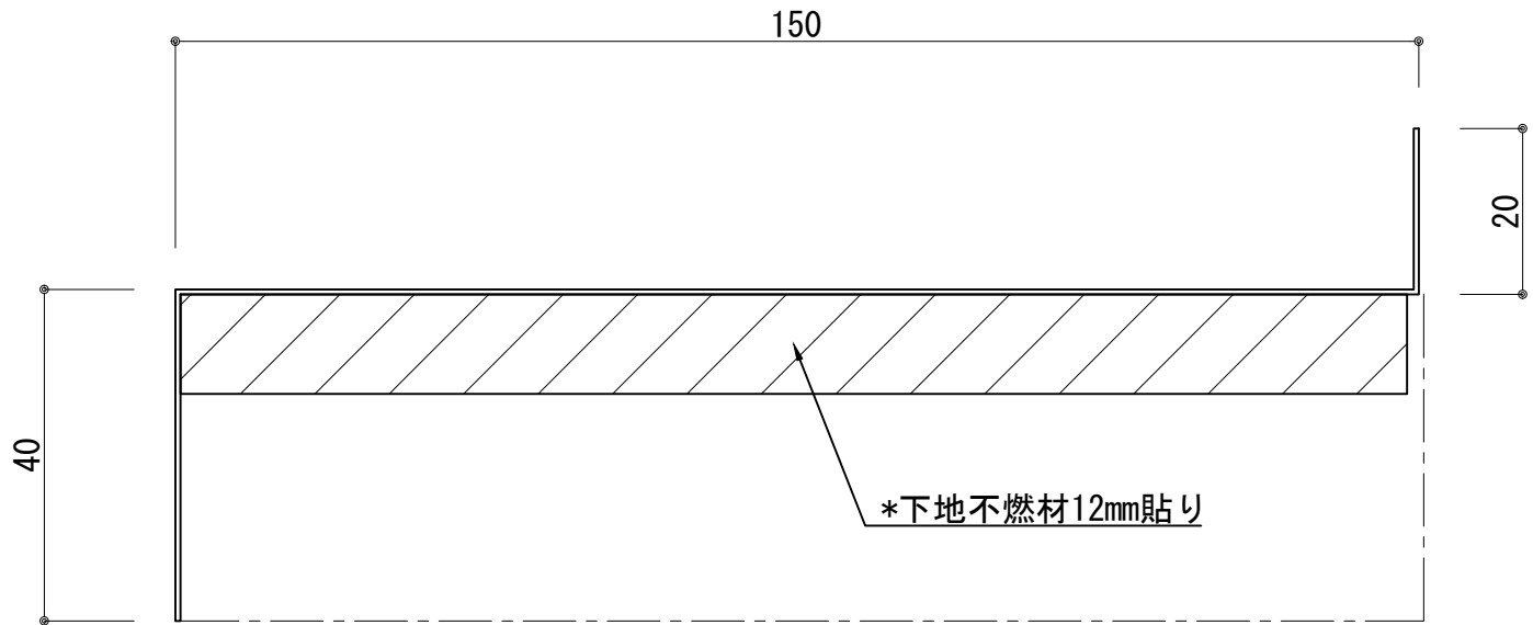
A-A'部断面図 1/1
